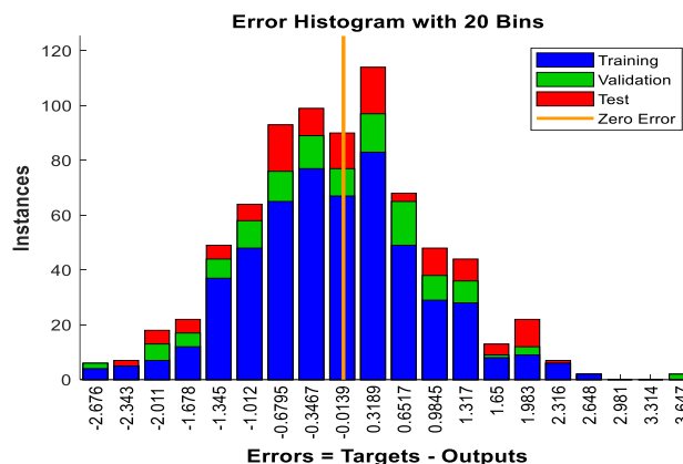
شکل ۴: میزان خطای شبکه عصبی
